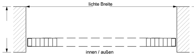
Montage in der Laibung, Gitterflügel feststehend
